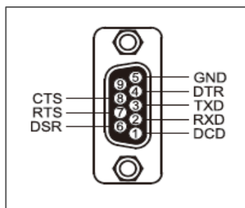
RS232 DB9 メス
