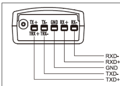
RS422 端子ブロック
