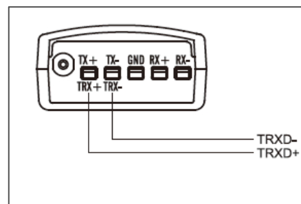
RS485 端子ブロック
