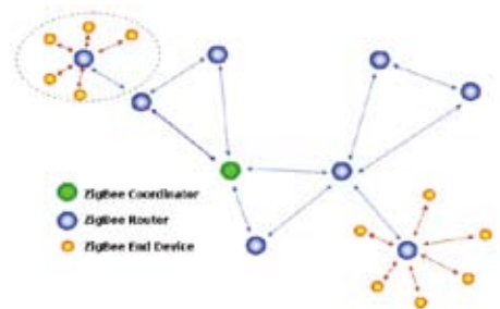
接続イメージ図
